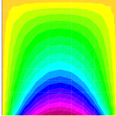
Solución generada con PLaplaceP1.edp usando plot
