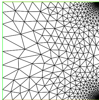
Malla final generada con PoissonReaccion-adap.edp
