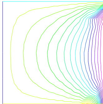
Solucion inicial obtenida con PoissonReaccion-adap.edp
