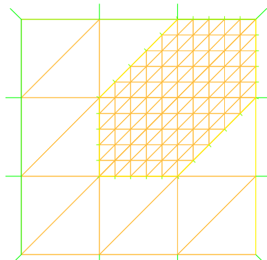
Soporte función de base 10 obtenido con base.edp
