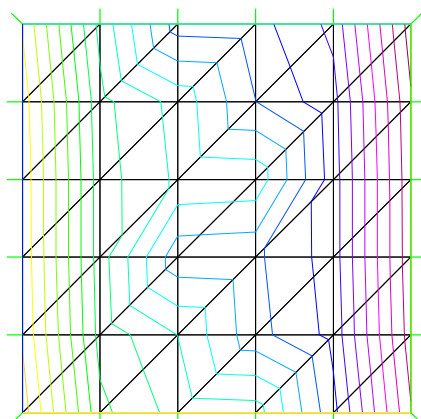
Malla y función inicial generada con Poisson-adap.edp
