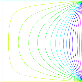
Solucion final obtenida con PoissonReaccion-adap.edp
