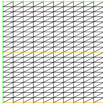
Dos mallas coincidentes en la interfaz generadas con ff13-ddm.edp
